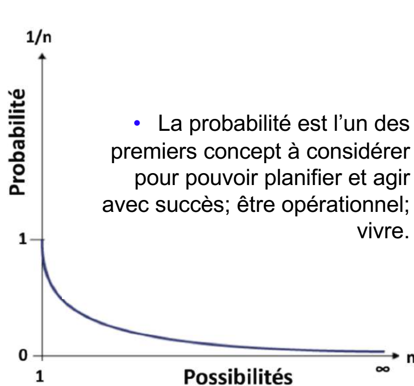
Fig. La probabilité d'un message spécifique diminue avec le nombre de possibilités
