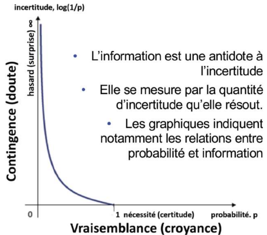
Fig. En fonction des variations de probabilité, des concepts contrastés se visitent: probabilité et incertitude, vraisemblance et contingence, chance et nécessité.
